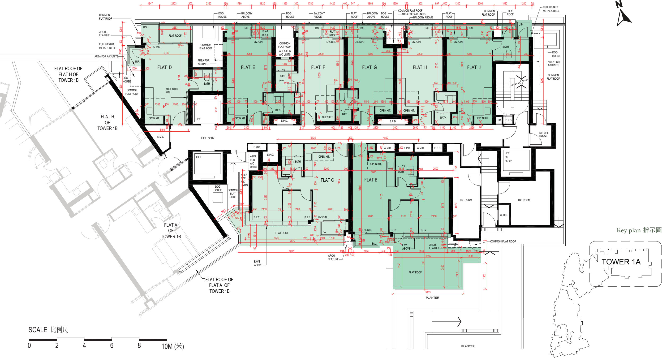
TOWER 1A 3/F (GARDEN FLOOR) FLOOR PLAN 第1A座 3樓(花園層)平面圖
