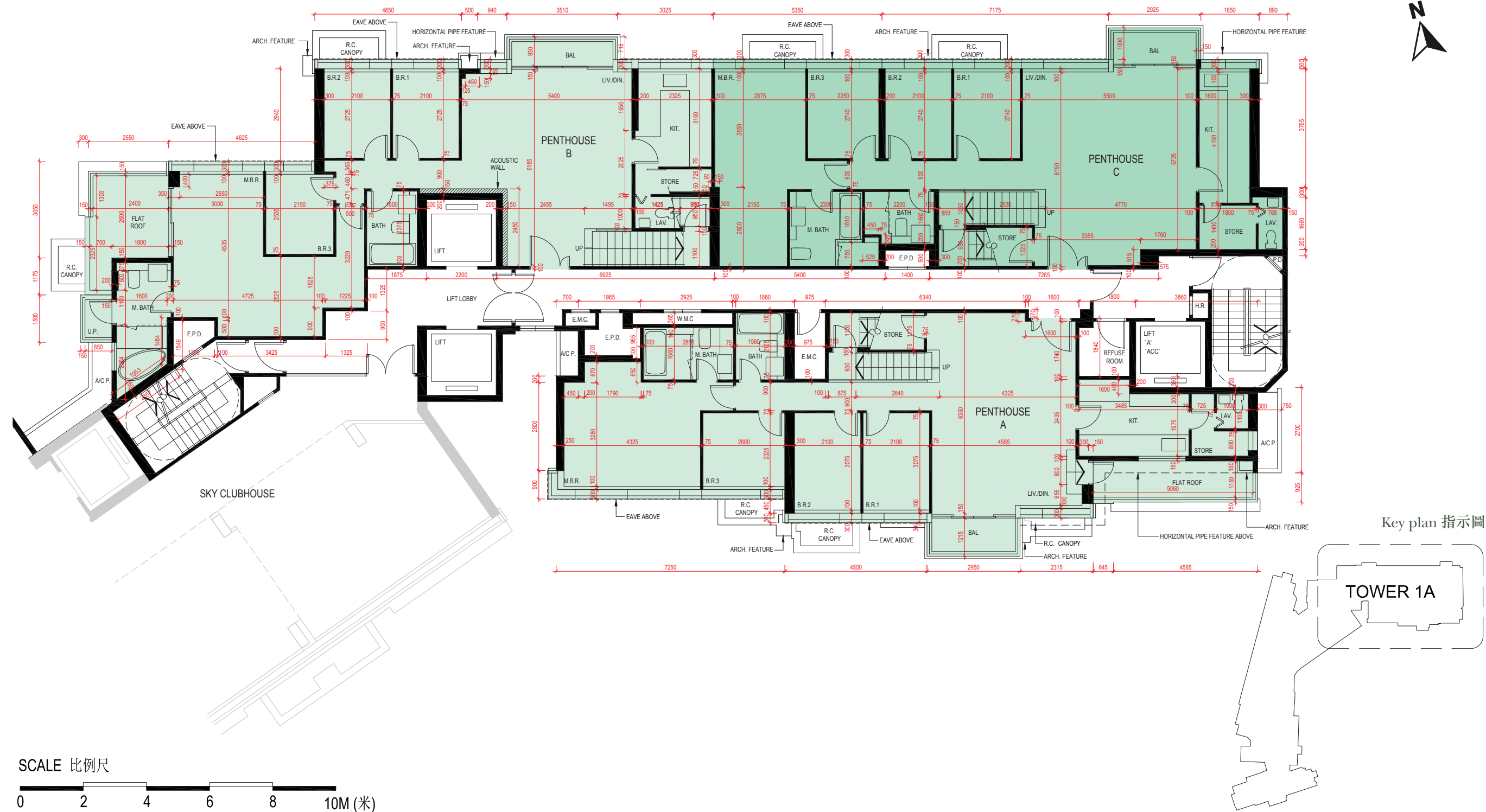
TOWER 1A 35/F PENTHOUSE FLOOR FLOOR PLAN 第1A座 35樓頂層平面圖
